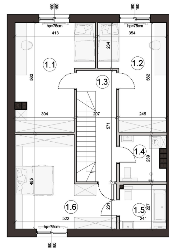
Rzut piętra
