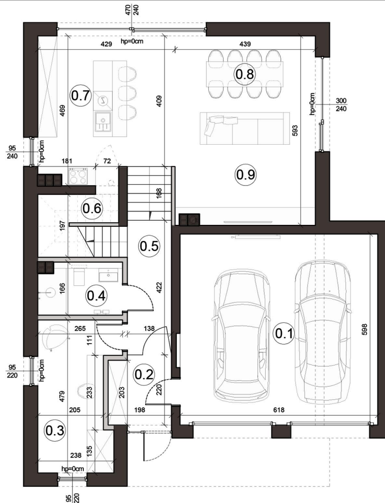
Rzut parteru
