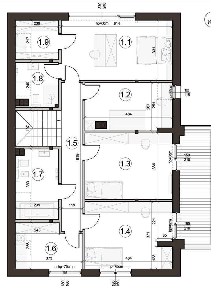
Rzut piętra
