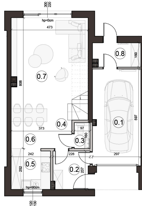
Rzut parteru
