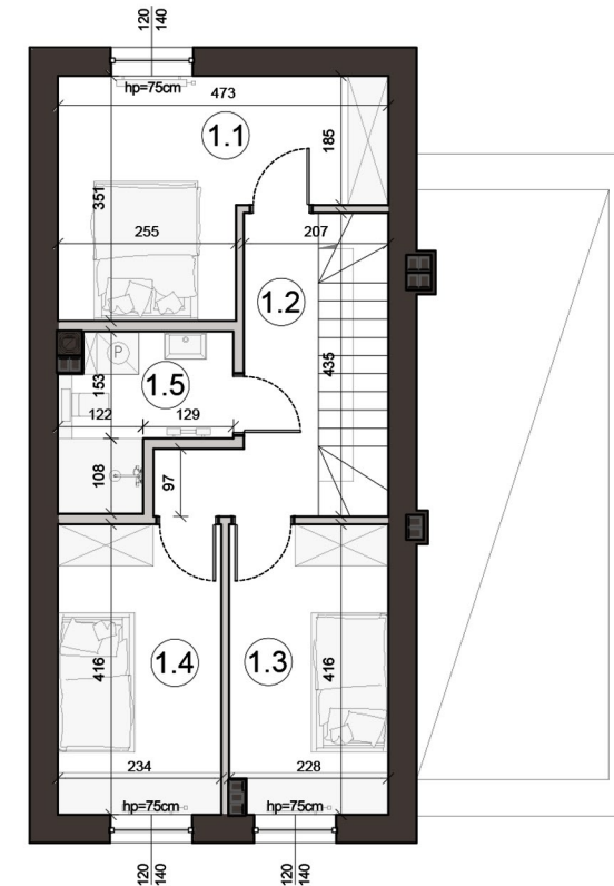
Rzut piętra
