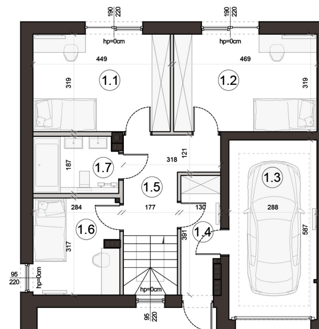
Rzut piętra
