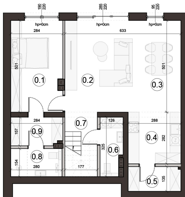
Rzut parteru
