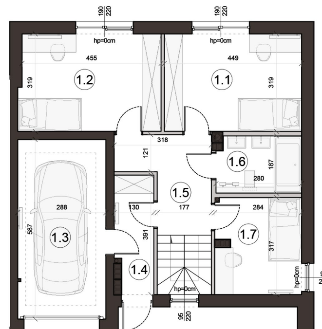
Rzut piętra
