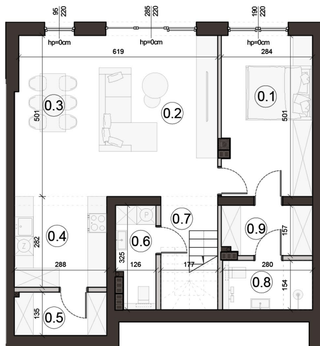
Rzut parteru
