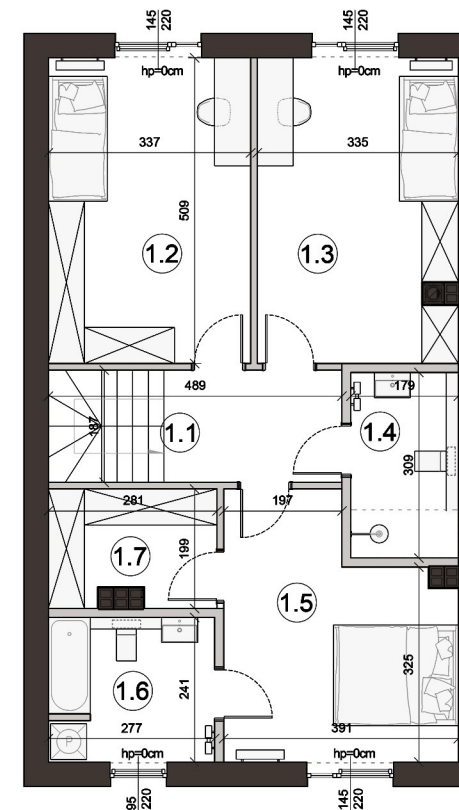
Rzut piętra
