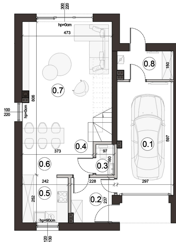
Rzut parteru
