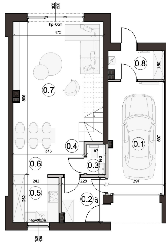
Rzut parteru
