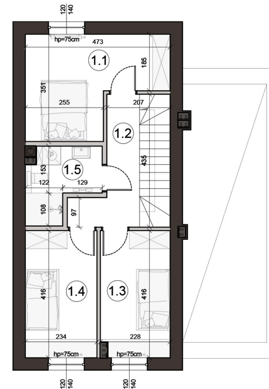
Rzut piętra
