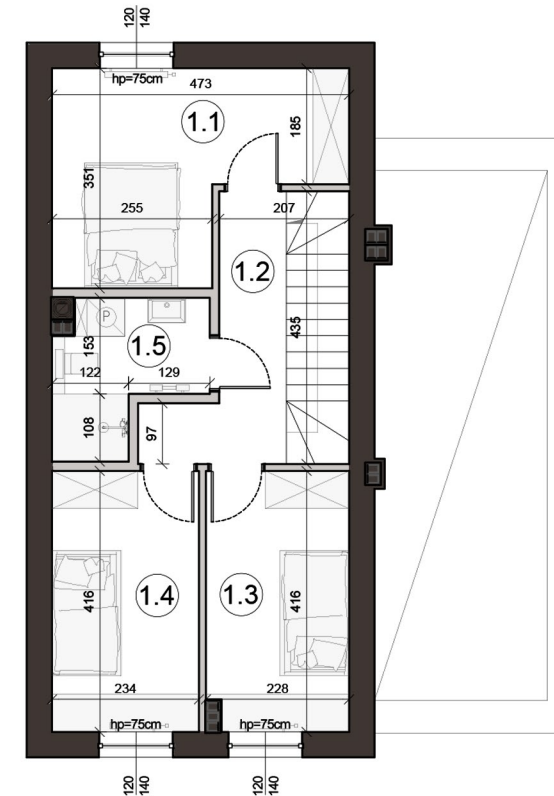
Rzut piętra
