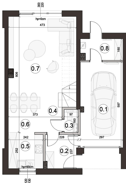
Rzut parteru
